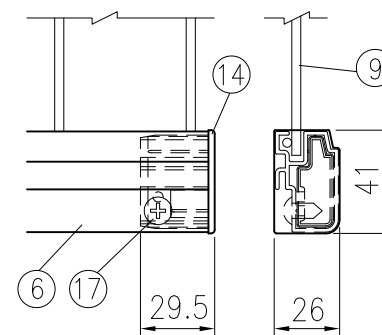
D 部詳細図 (1/3)
