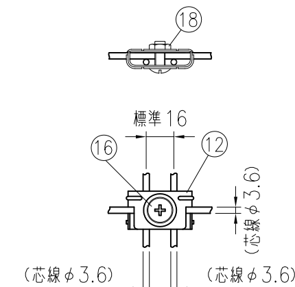
I 部詳細図 (1/3)
