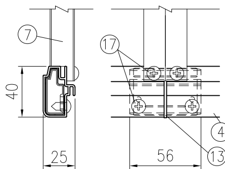
F 部詳細図 (1/3)
