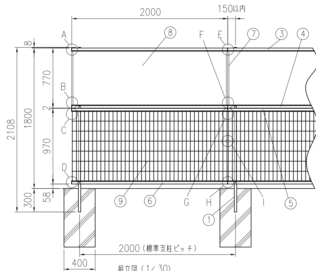
組立図 (1/30)
