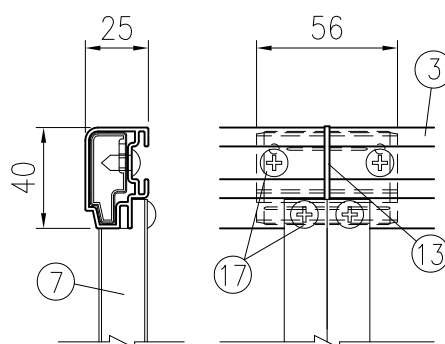
E 部詳細図 (1/3)
