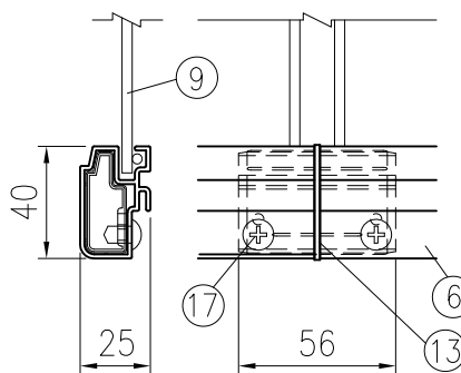
H 部詳細図 (1/3)
