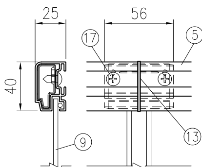
G 部詳細図 (1/3)
