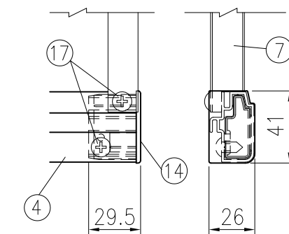
B 部詳細図 (1/3)
