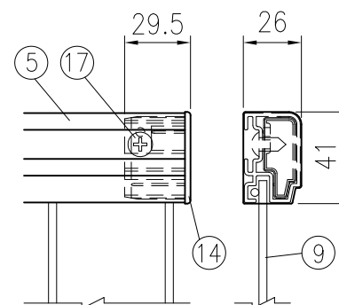
C 部詳細図 (1/3)
