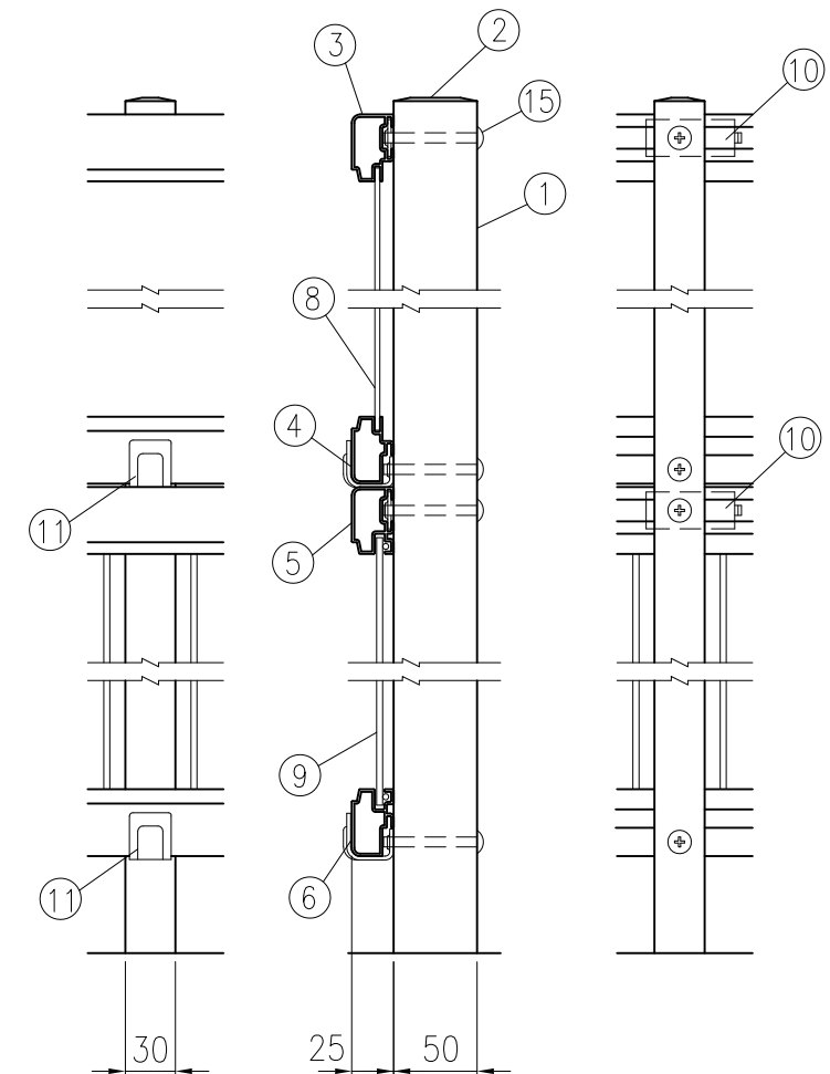
取付部詳細図 (1/5)
