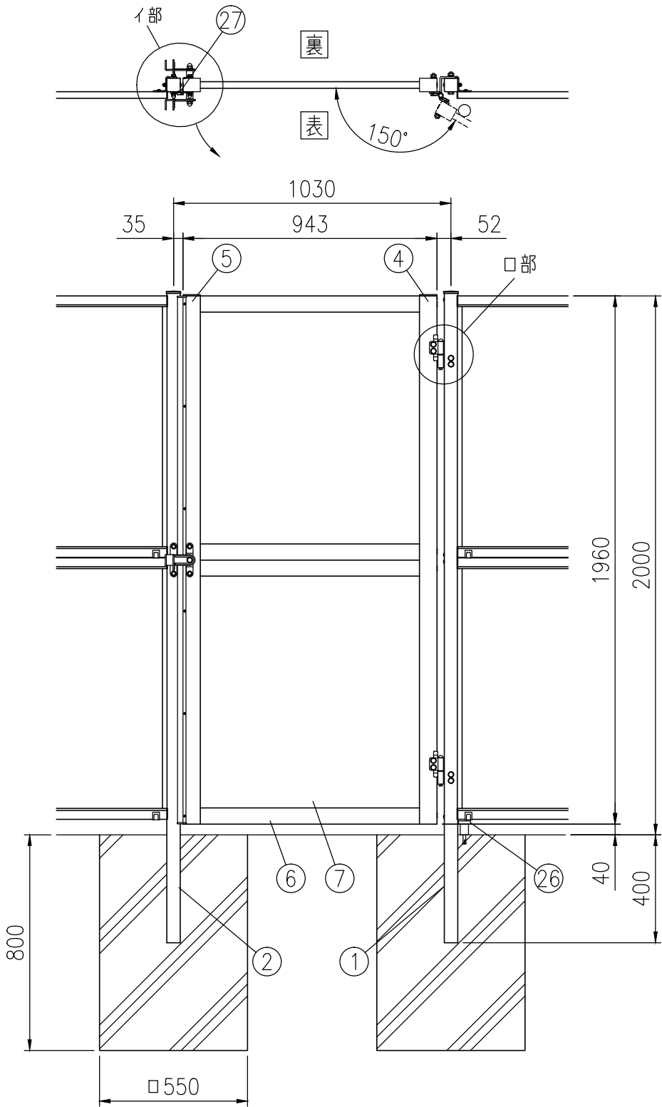
組立図 （1／20）
