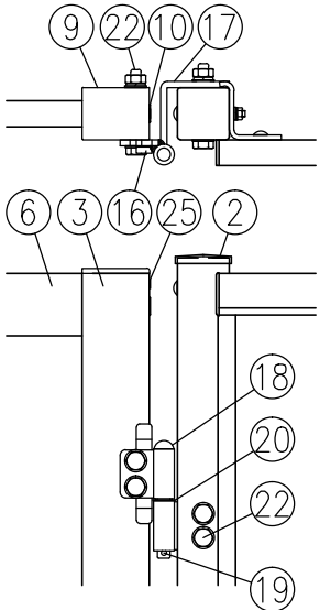
ロ部詳細図（1／8）
