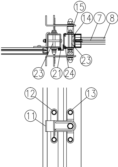
イ部詳細図（1／8）
