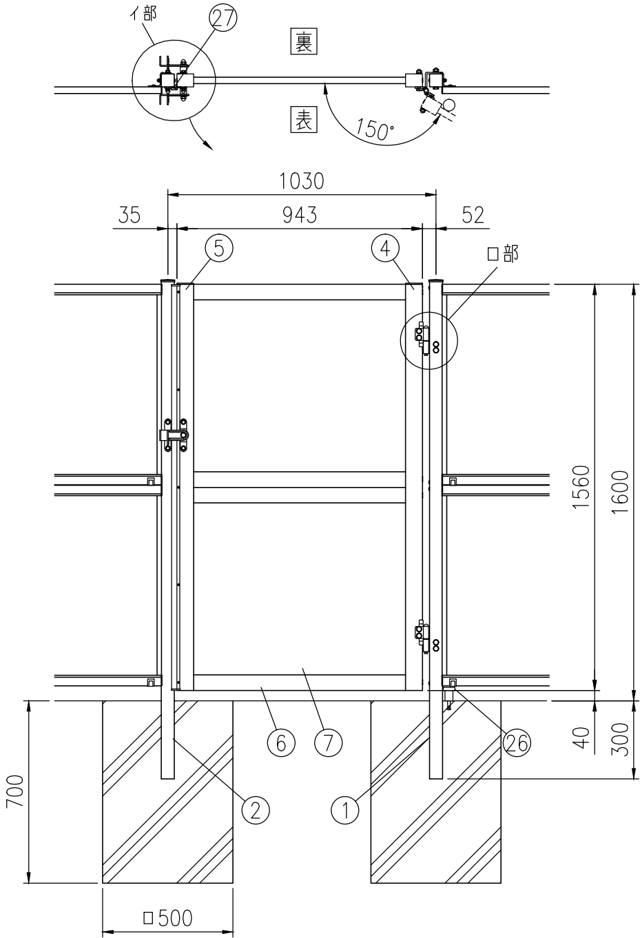
組立図 （1／20）
