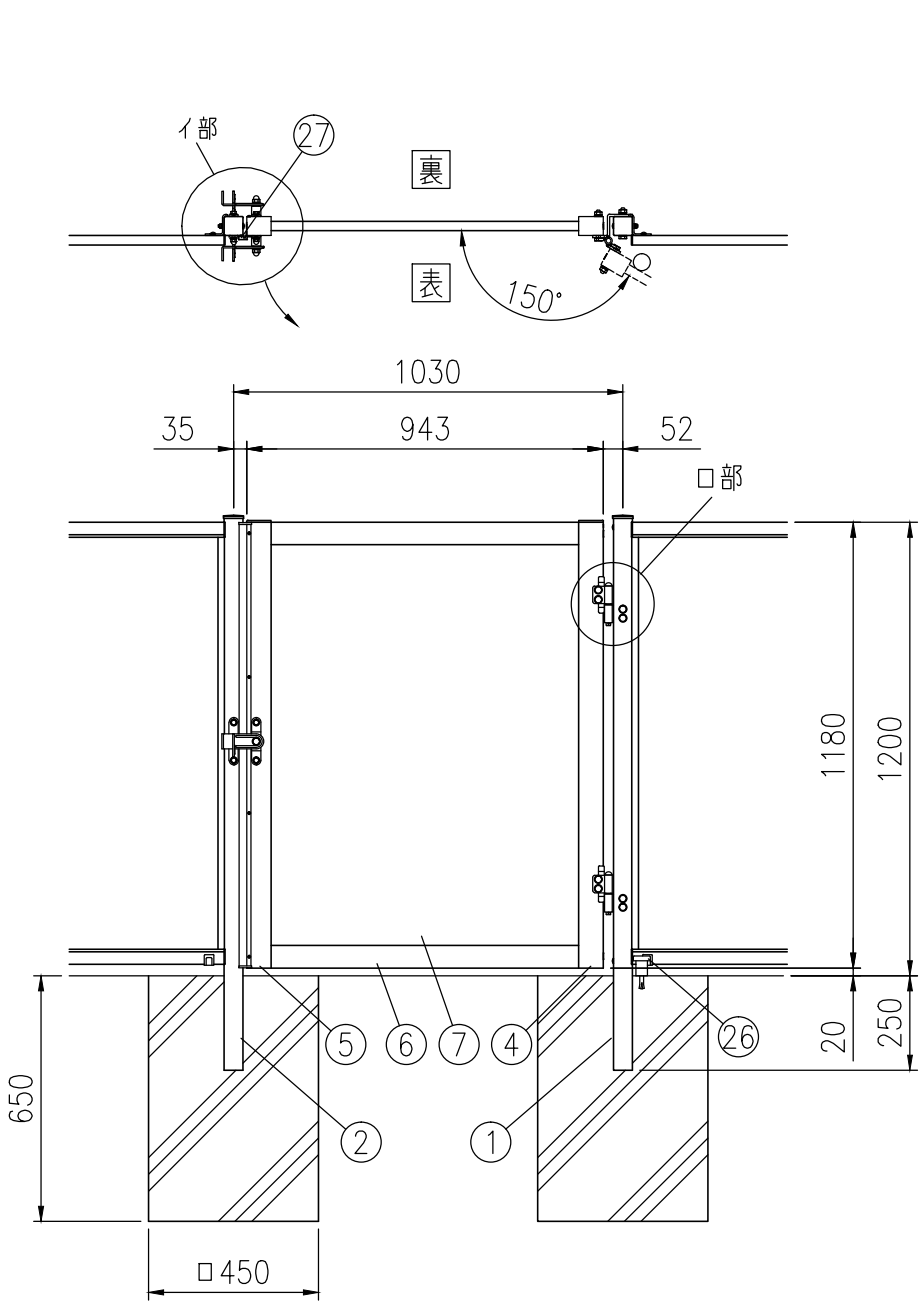
組立図 （1／20） 吊元右側、表開きの時 注）基礎の大きさは参考寸法です。
