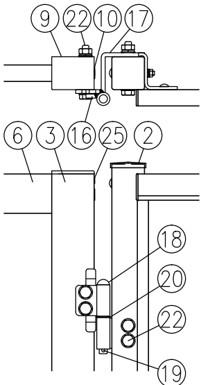
K部詳細図 (1/8)
