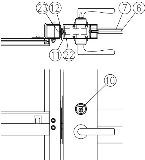
イ部詳細図 (1/8)
