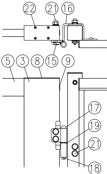
ロ部詳細図 (1/8)
