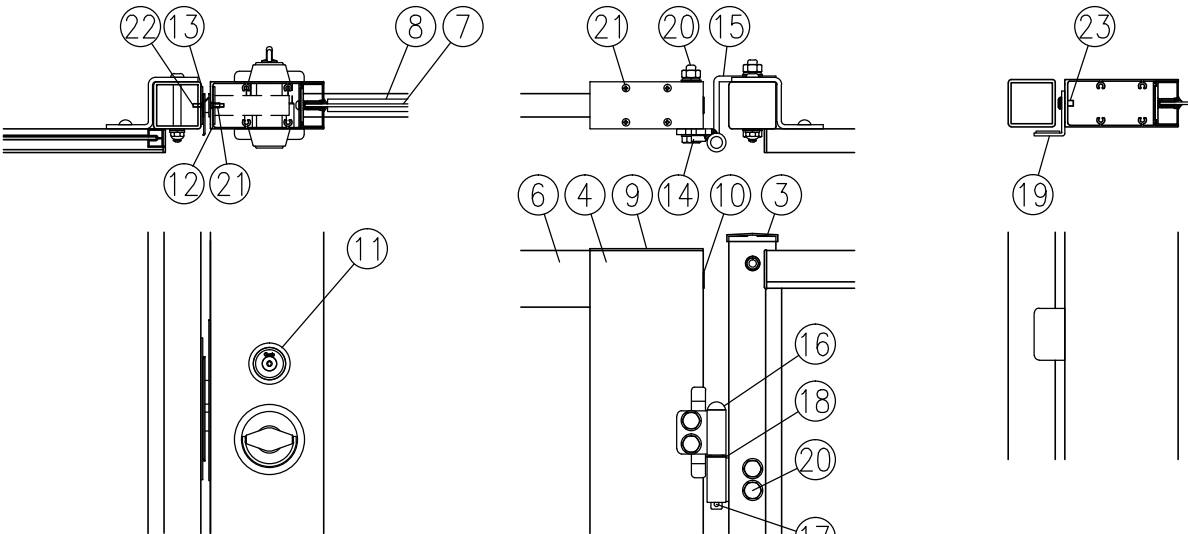
イ部詳細図 (1/8)
