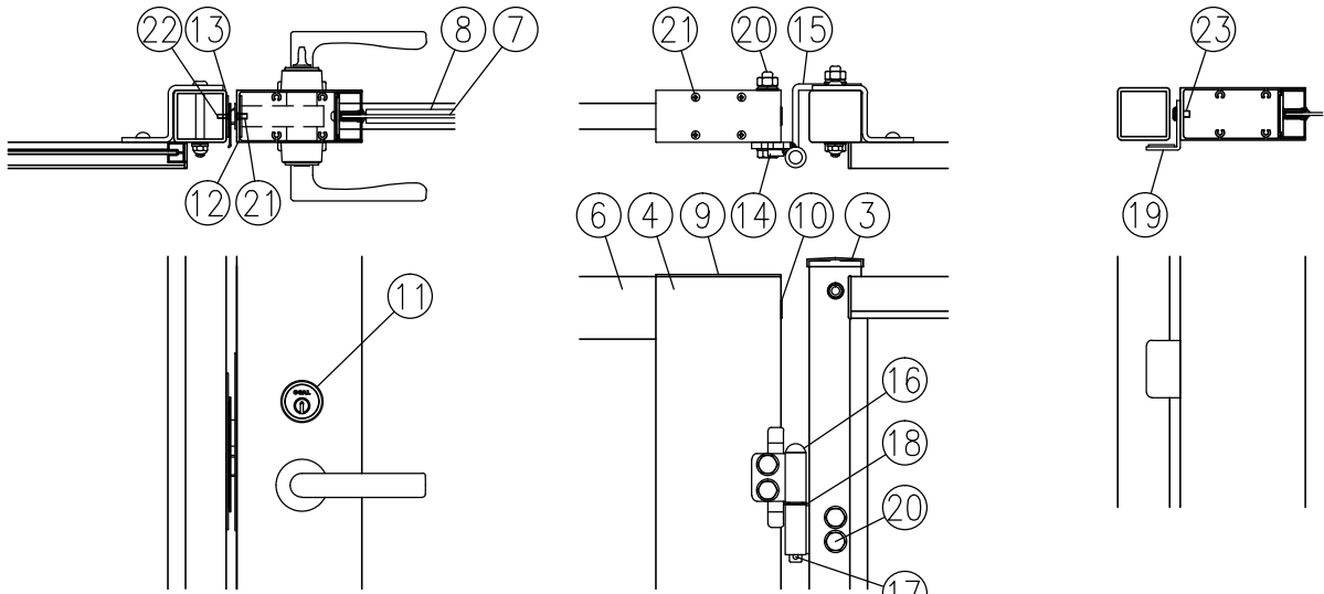
イ部詳細図（1/8）
