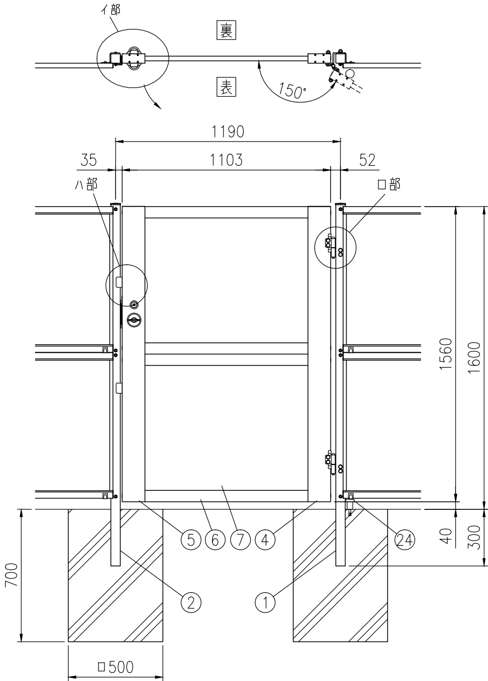
組立図 (1/20)
