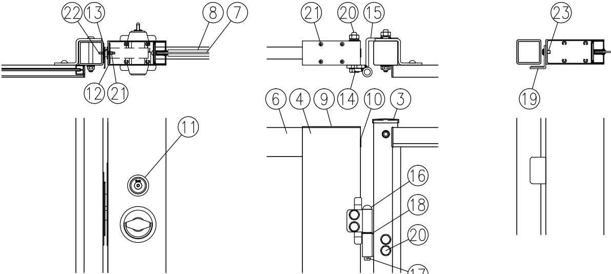
イ部詳細図（1/8） ロ部詳細図（1/8） ハ部詳細図（1/8）
