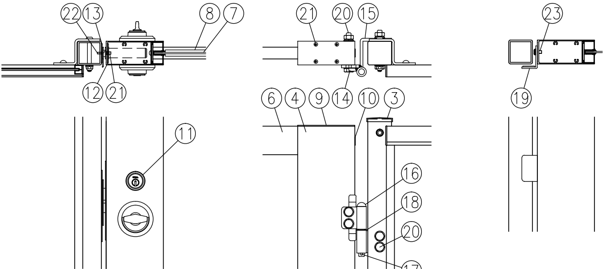
イ部詳細図（1/8）
