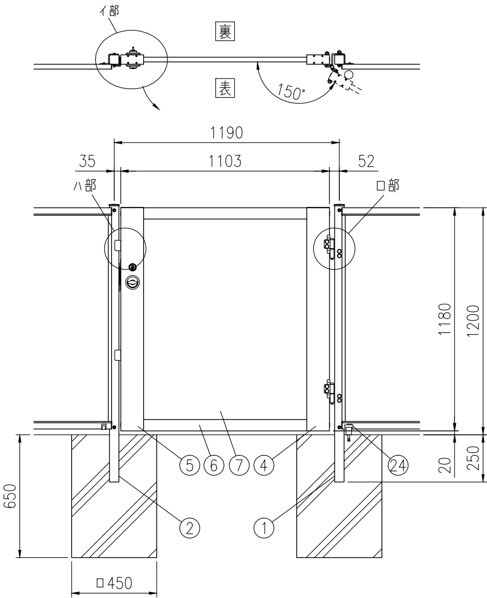
組立図（1/20）
