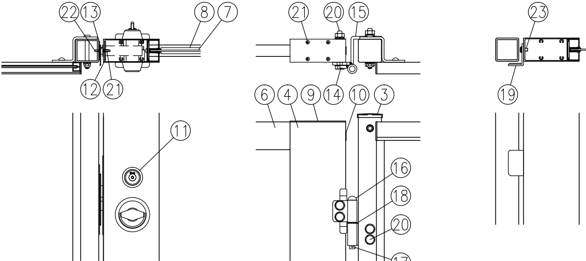
イ部詳細図（1/8）
