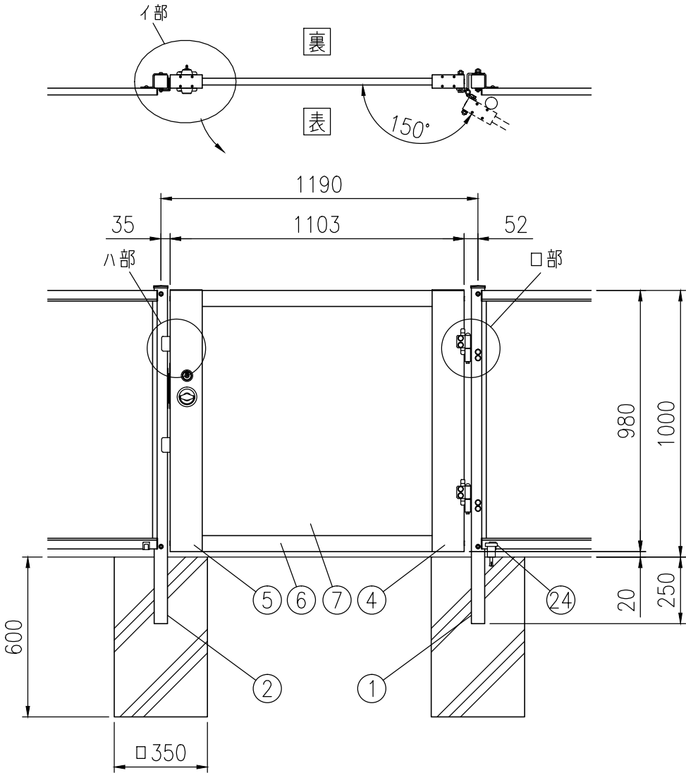
組立図（1/20）
