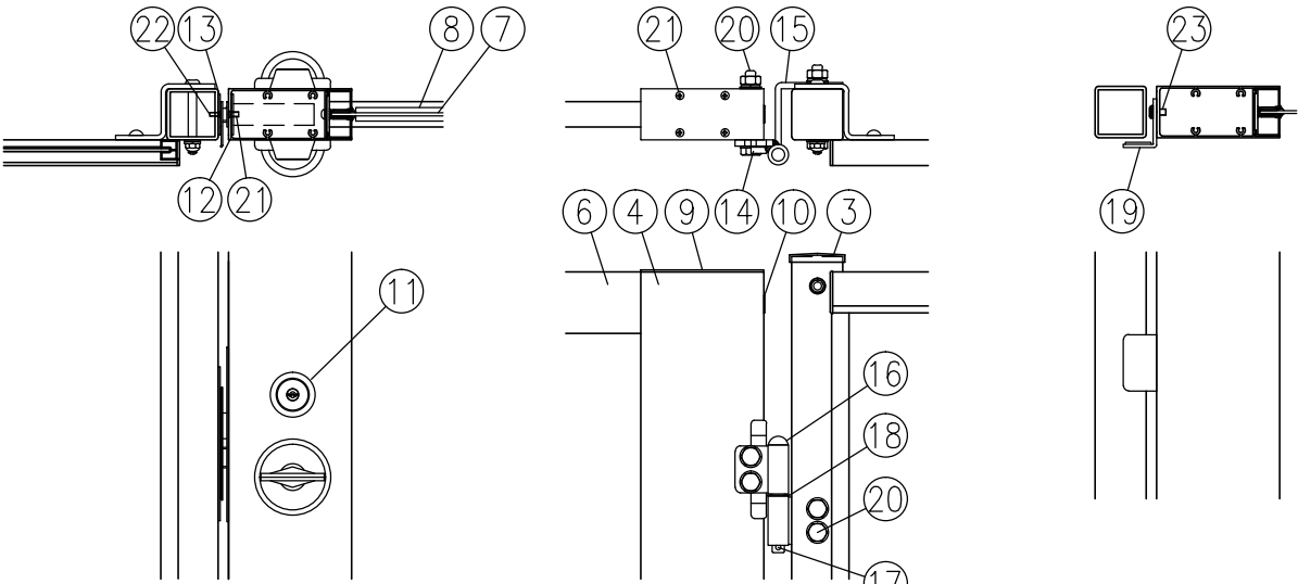
イ部詳細図 (1/8)
