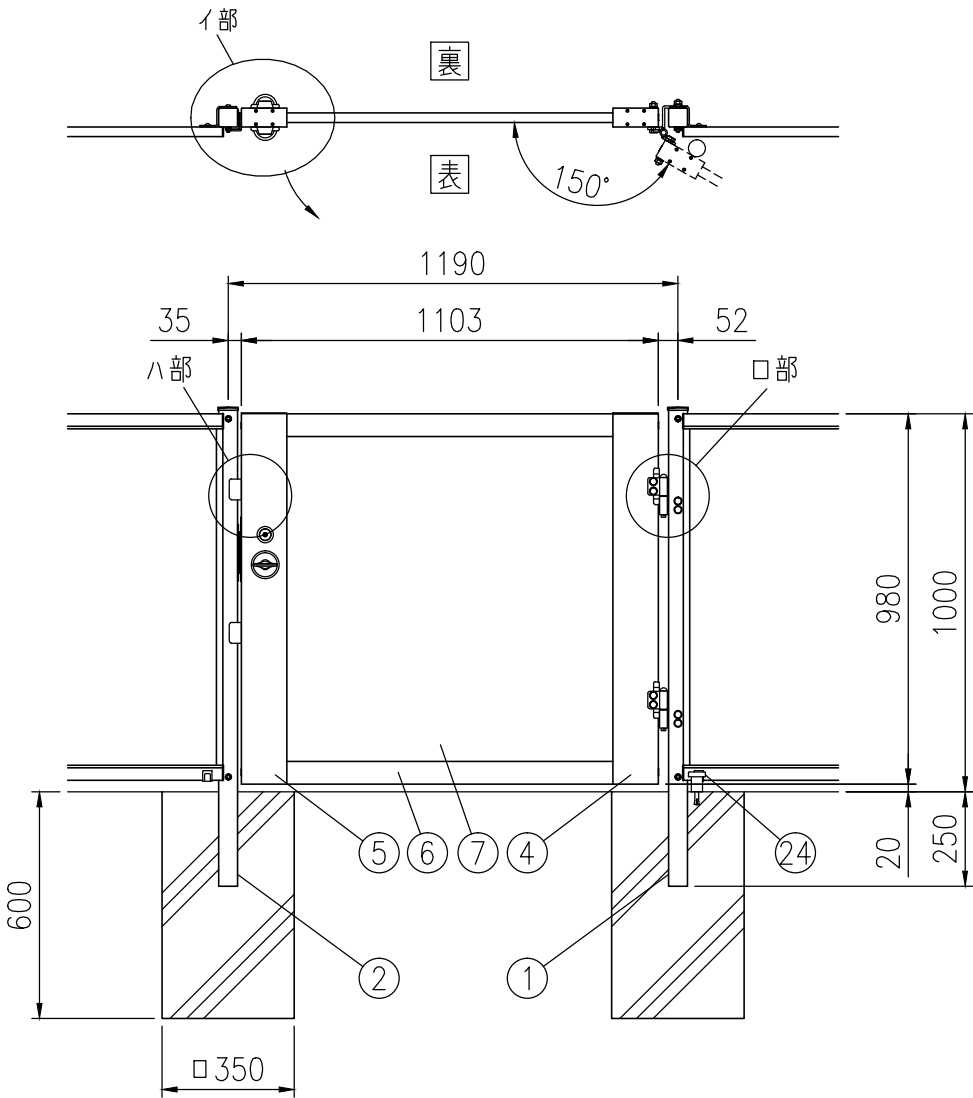
組立図 (1/20)
