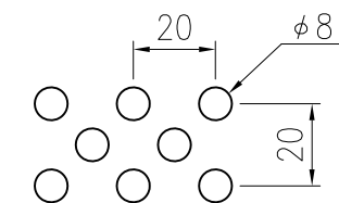
パンチング詳細図 (1/2)
