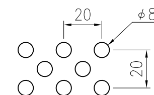
パンチング詳細図 (1/2)
