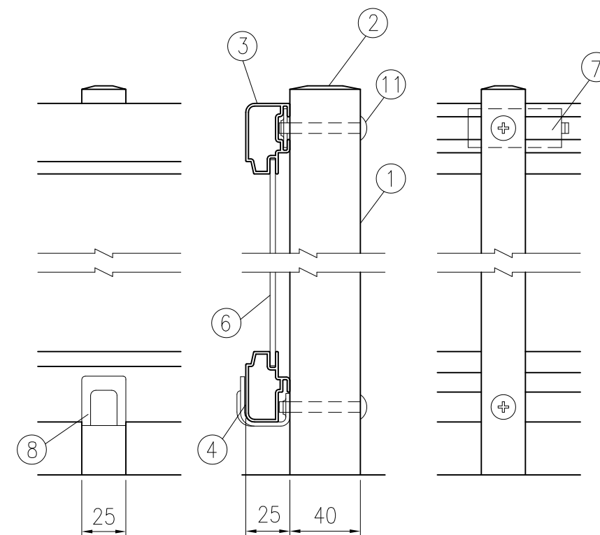
取付部詳細図 (1/3)
