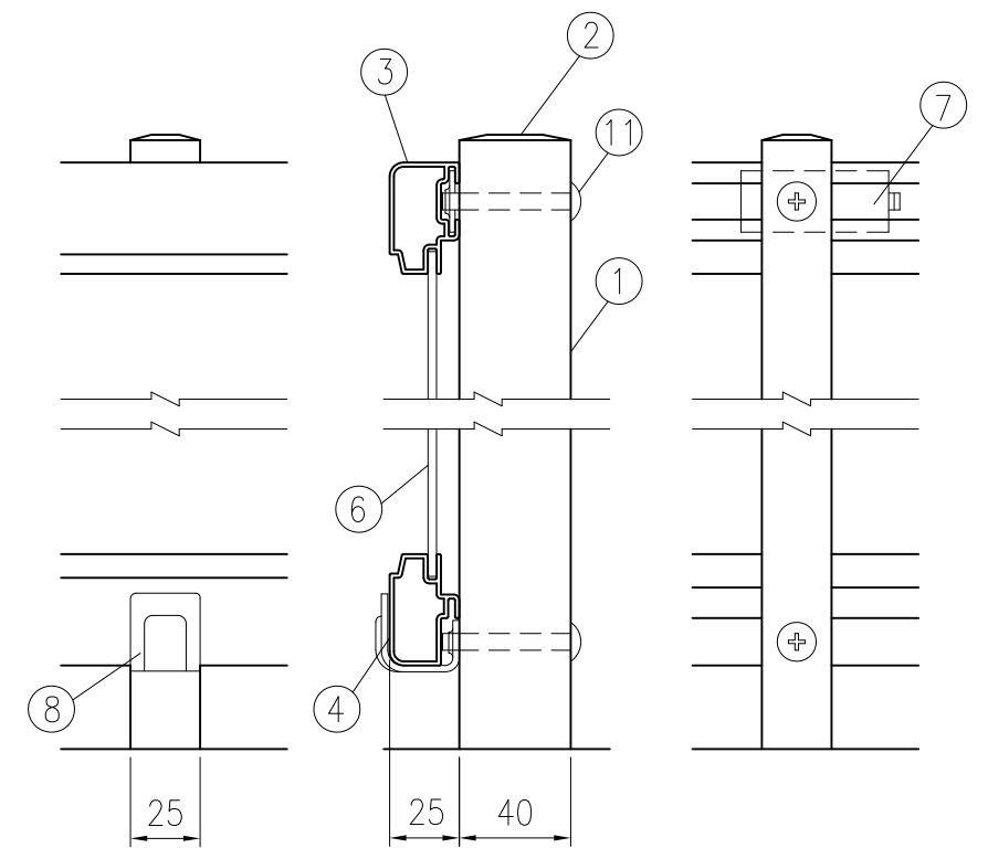
取付部詳細図 (1/3)
