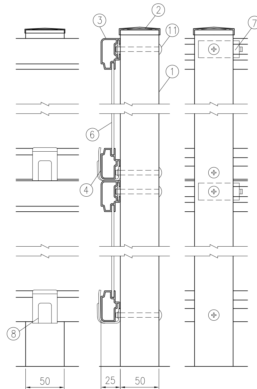
取付部詳細図 (1/3)
