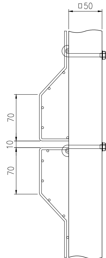
上下パネル部詳細図 (1/3)
