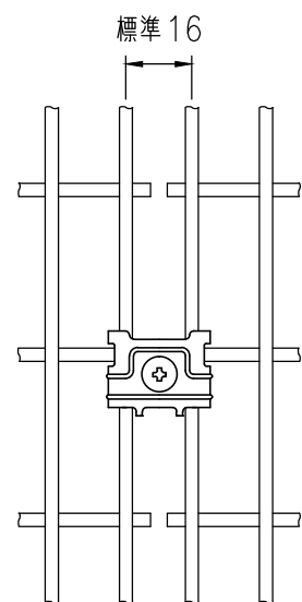
接続金具詳細図 (上部、中部) (1/2)
