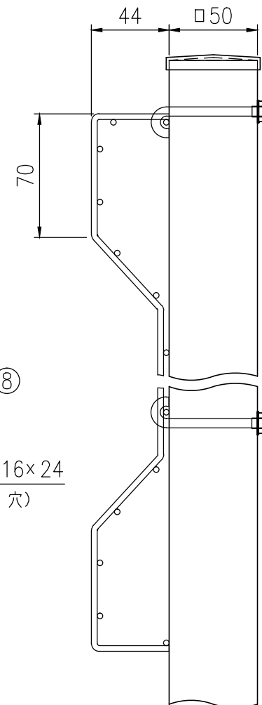
取付部詳細図 (1/3)
