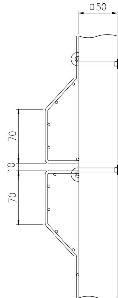
上下パネル部詳細図 (1/3)
