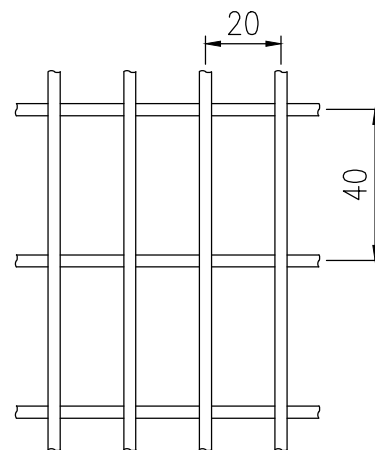
パネルマス目詳細図 (下部) (1/2)
