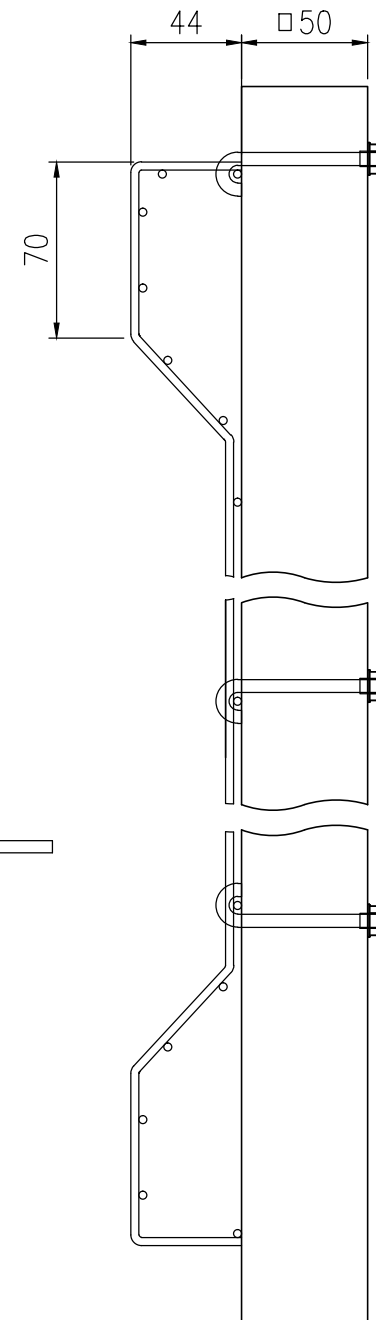
取付部詳細図 (1/3)
