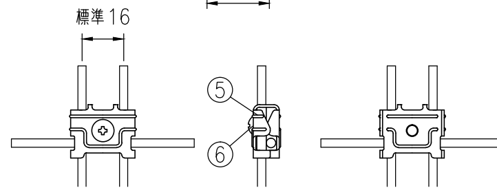
接続金具詳細図 (1/2)
