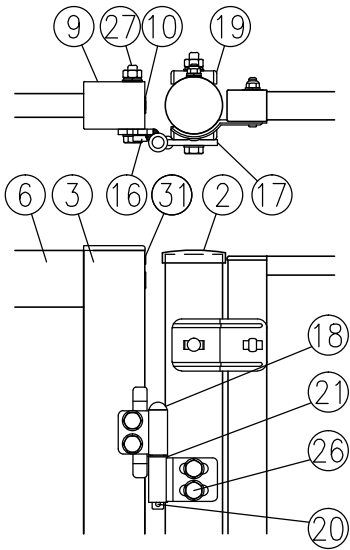
ロ部詳細図 (1/8)
