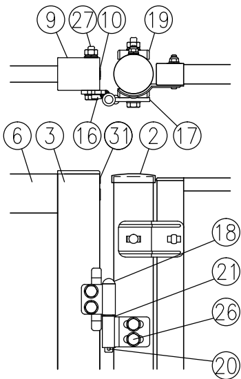
□部詳細図（1／8）
