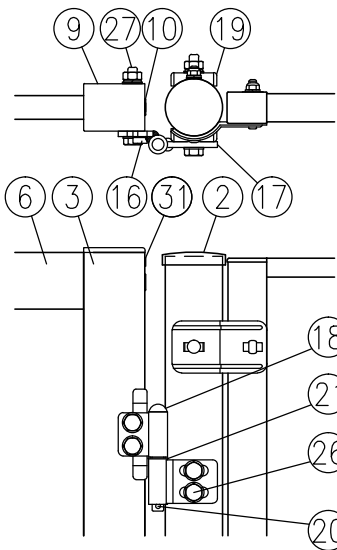
□部詳細図 (1/8)
