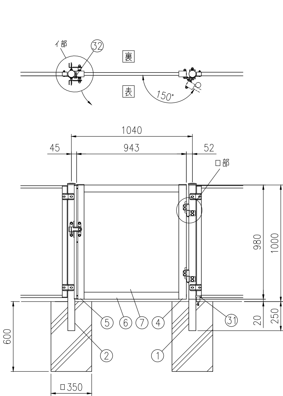
組立図（1/20）
