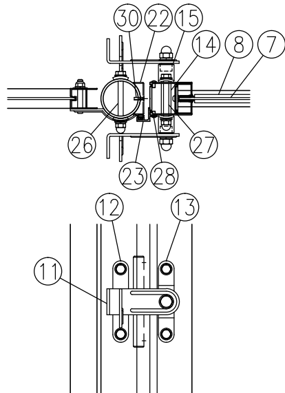
イ部詳細図（1/8）
