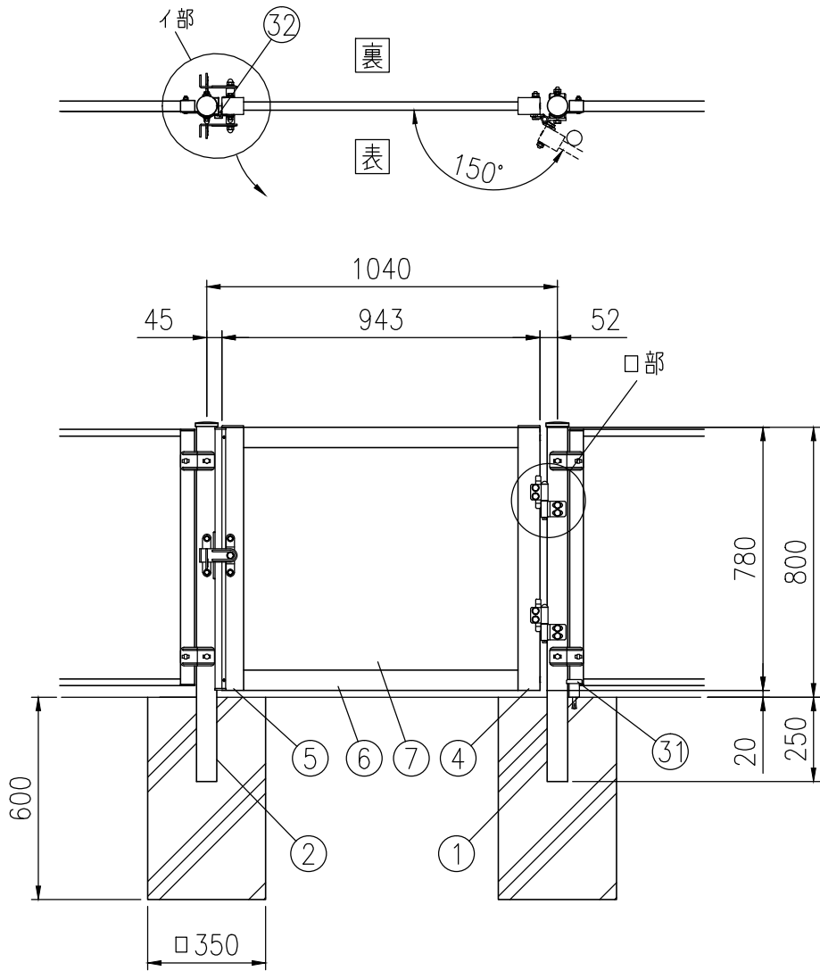
組立図（1/20）
