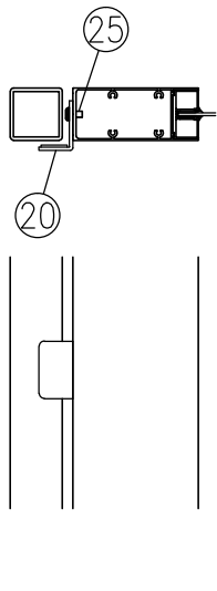
ハ部詳細図 (1/8)
