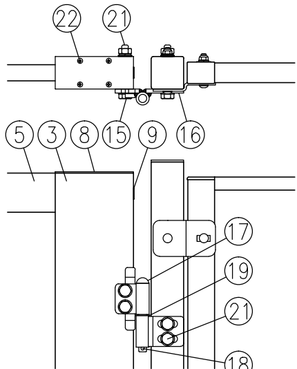
ロ部詳細図 (1/8)
