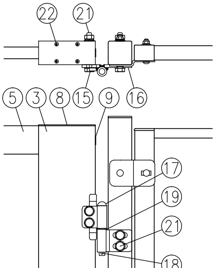
ロ部詳細図 (1/8)
