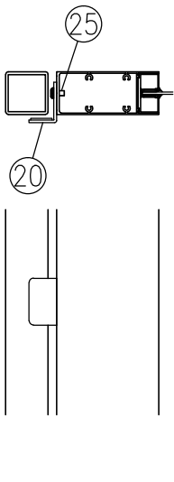
ハ部詳細図 (1/8)
