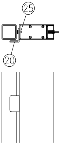
ハ部詳細図 (1/8)
