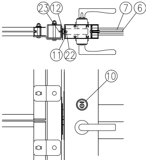
イ部詳細図 (1/8)
