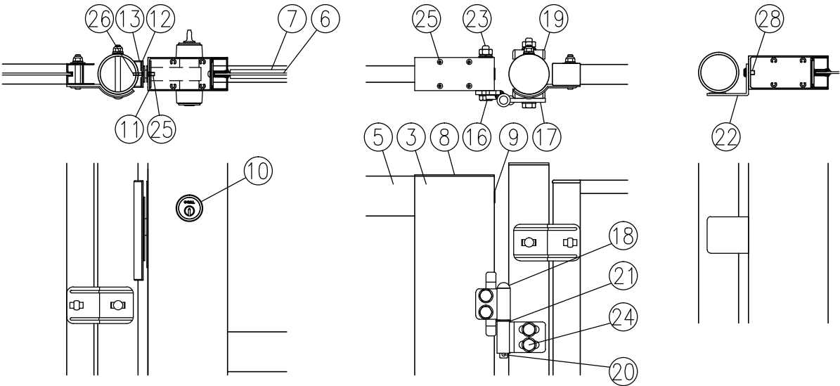
イ部詳細図（1/8）
