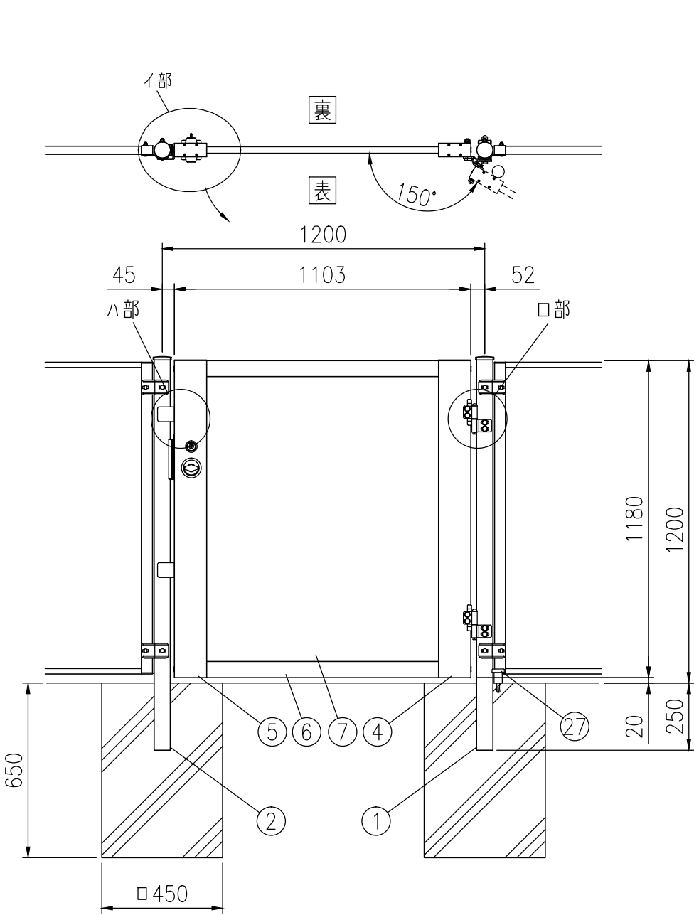
組立図 (1/20)
