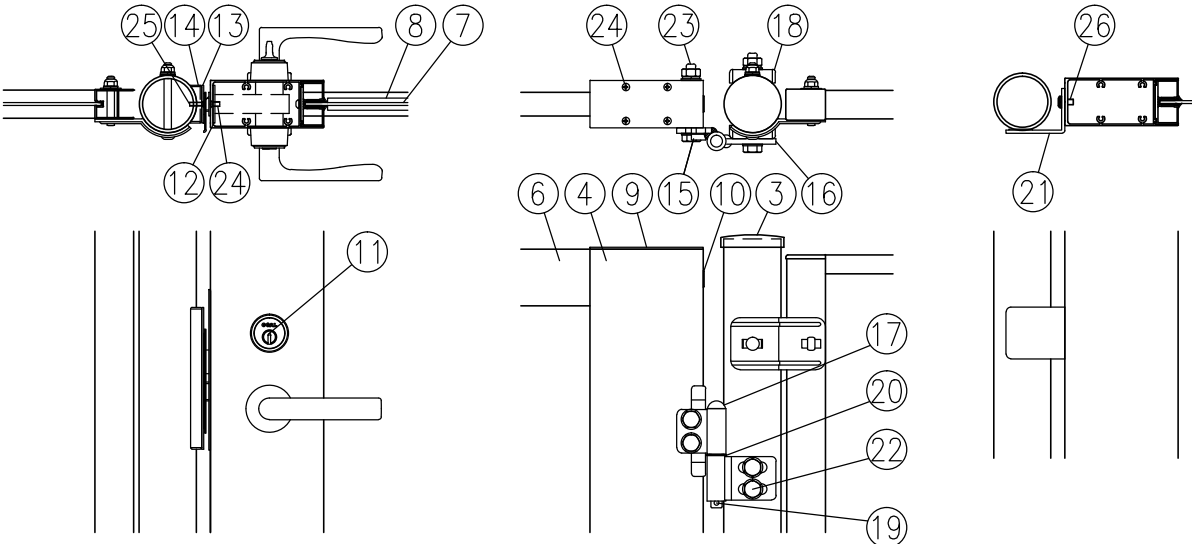
イ部詳細図（1/8）
