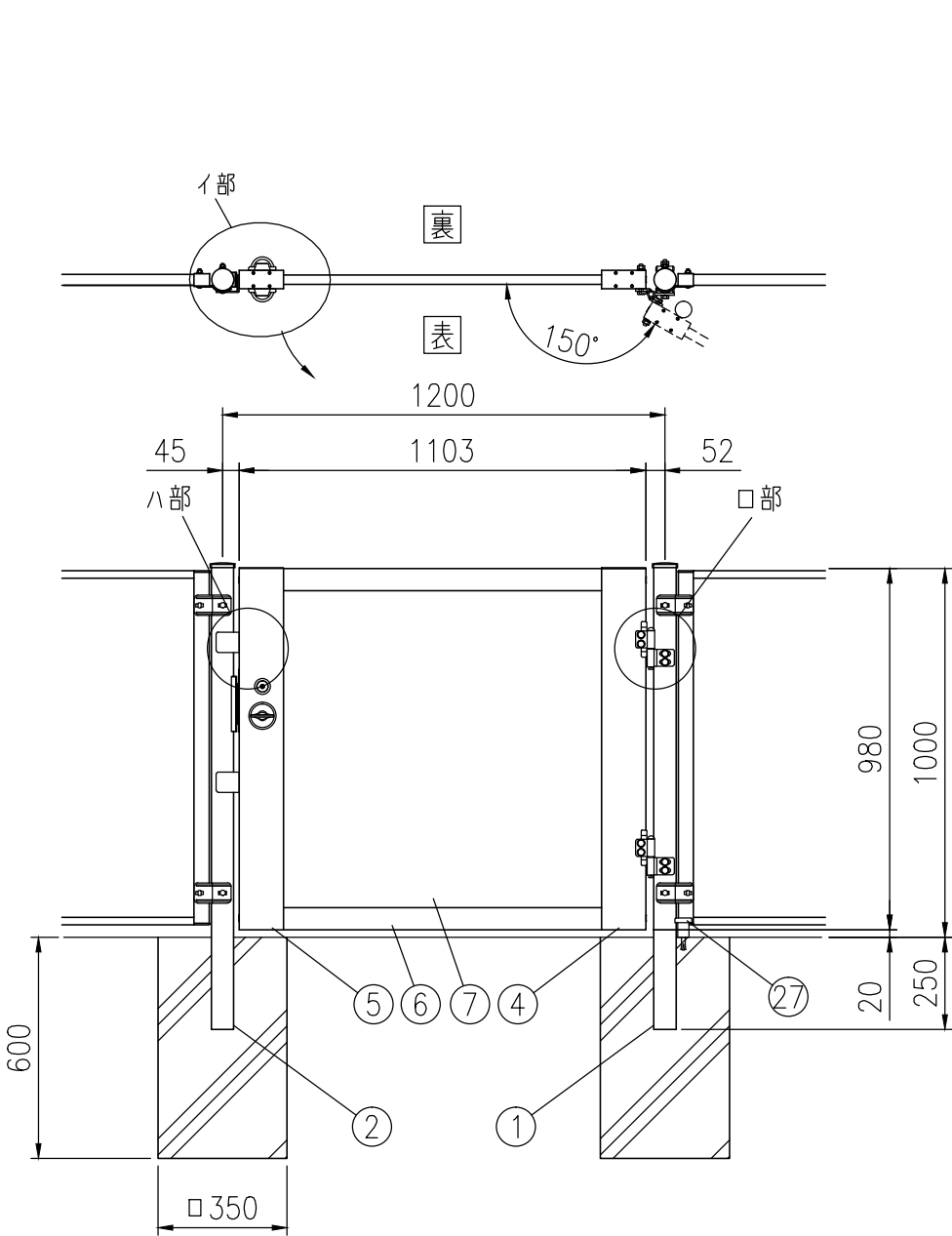
組立図（1/20）
