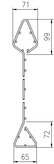
本体パネル詳細図 (1/5)
