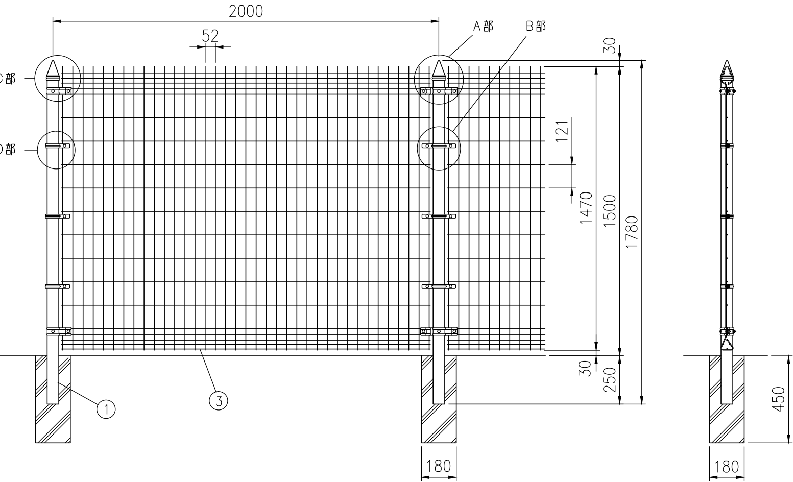
組立図 (1/20) 注) 基礎の大きさは参考寸法です。
