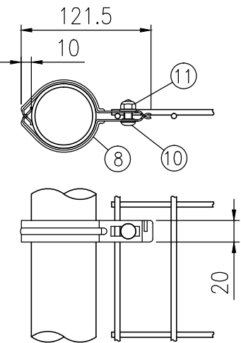
D部詳細図 (1/5)
