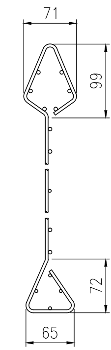
本体パネル詳細図 (1/5)
