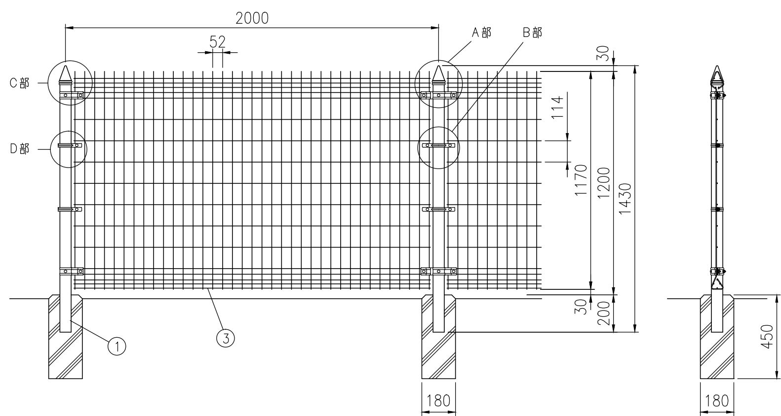
組立図 (1/20) 注) 基礎の大きさは参考寸法です。
