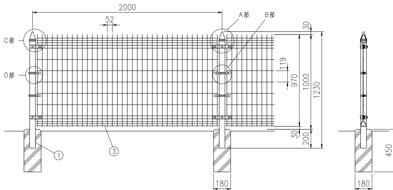
組立図 (1/20) 注) 基礎の大きさは参考寸法です。
