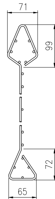
本体パネル詳細図 (1 / 5)
