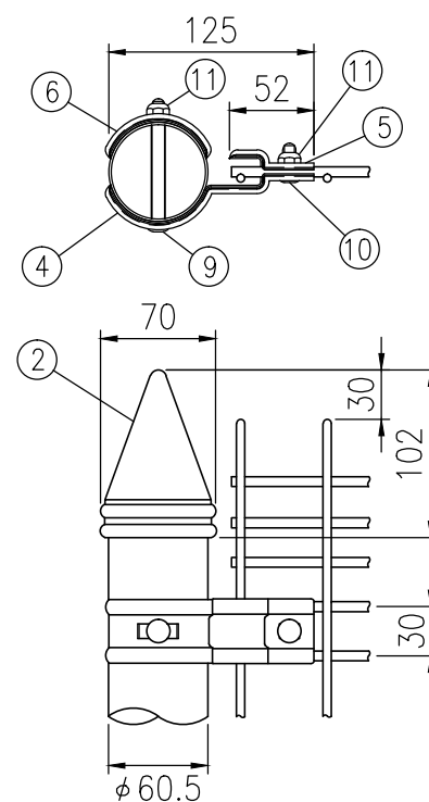
C部詳細図 (1 / 5)
