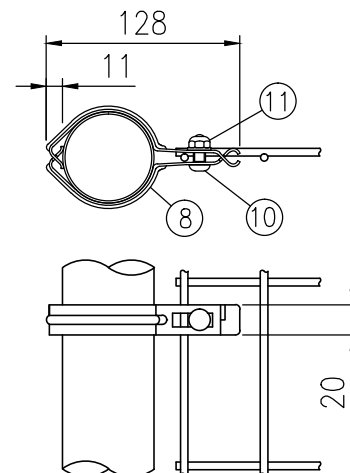
D部詳細図 (1 / 5)
