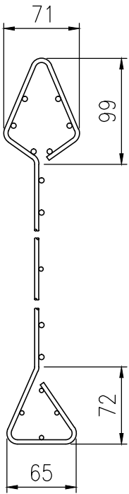
本体パネル詳細図 (1/5)
