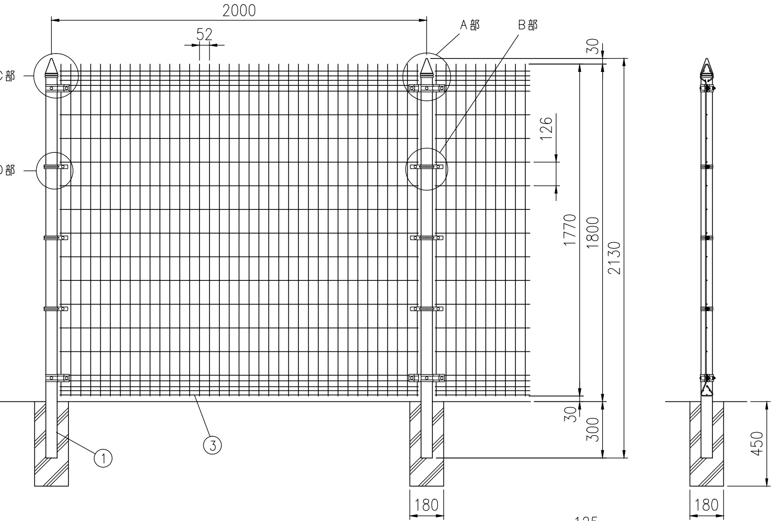
組立図 (1/20) 注) 基礎の大きさは参考寸法です。
