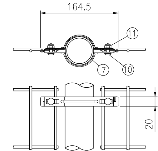
B部詳細図 (1/5)
