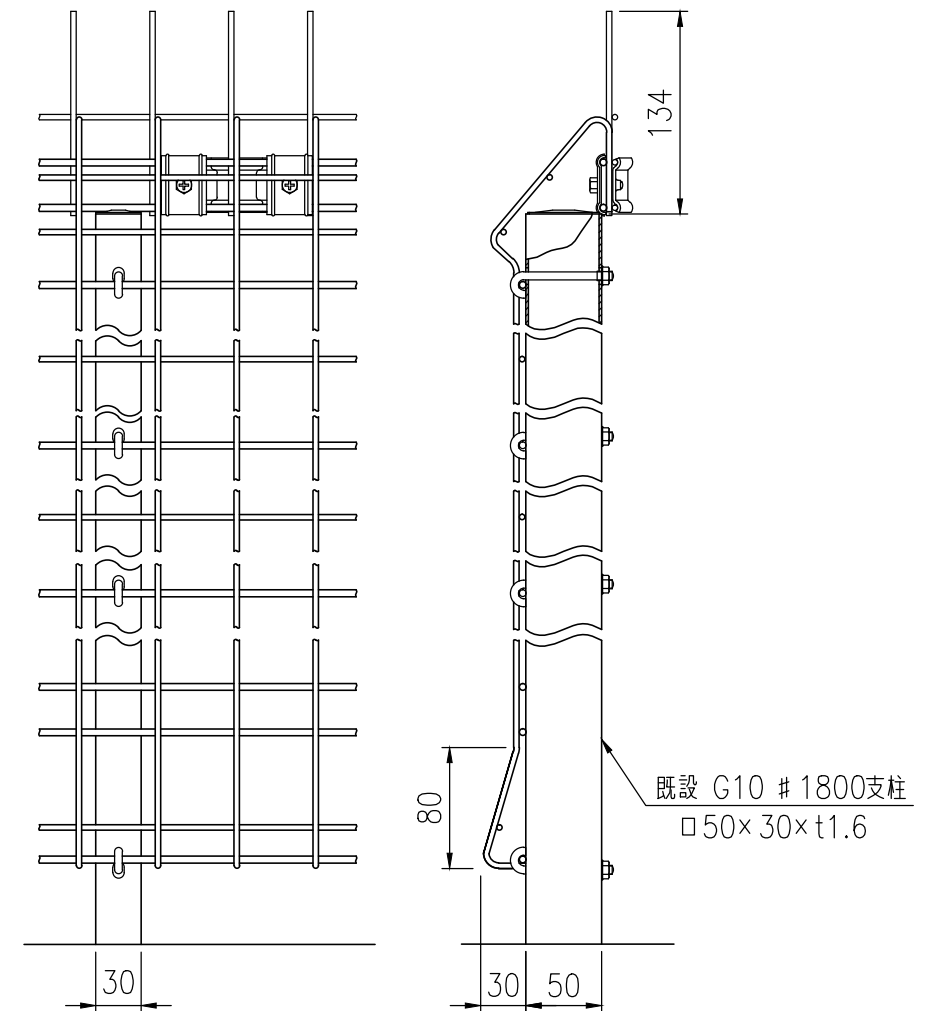
取付部詳細図 (1/5)
