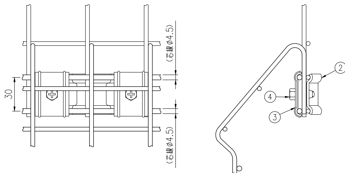
取付金具詳細図 (1/2)
