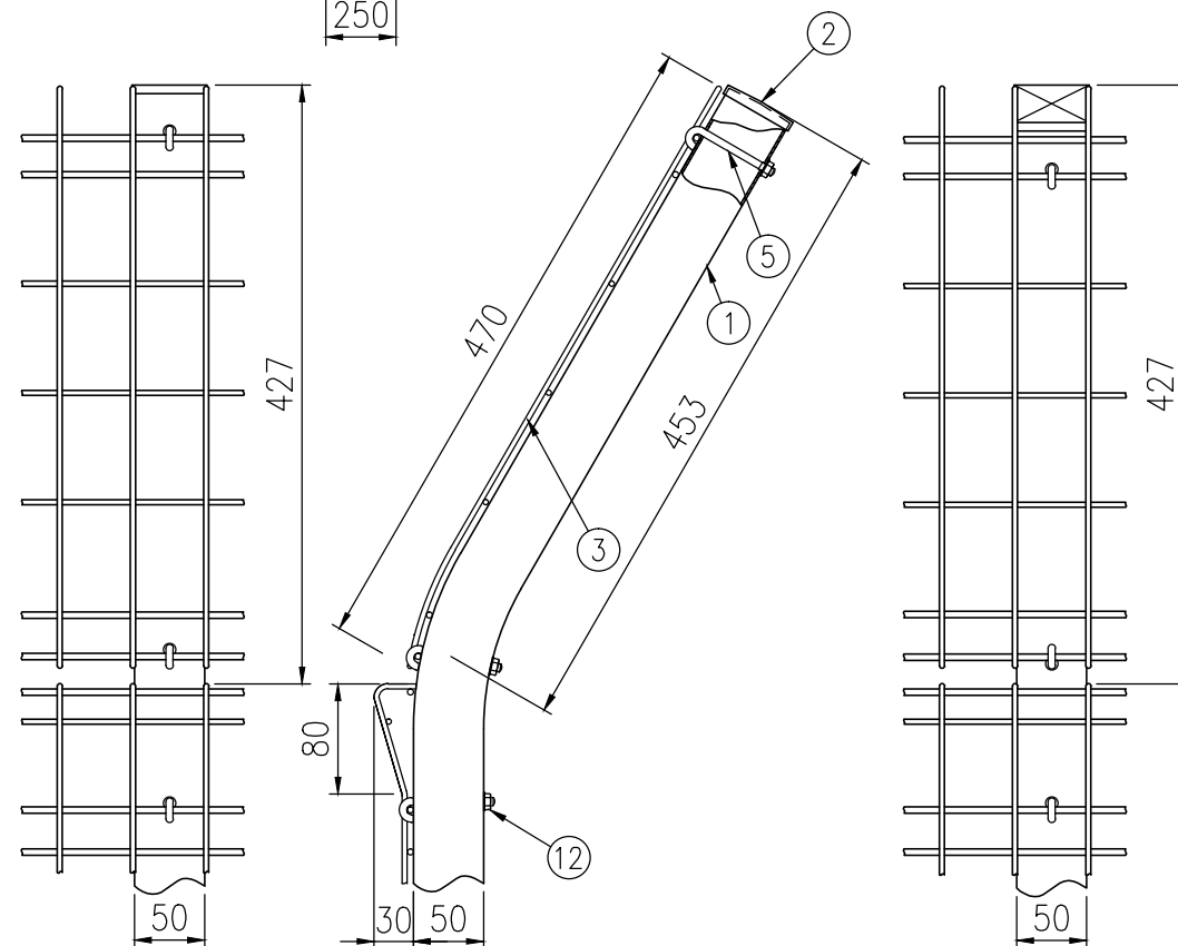
取付部詳細図 (1/6)
