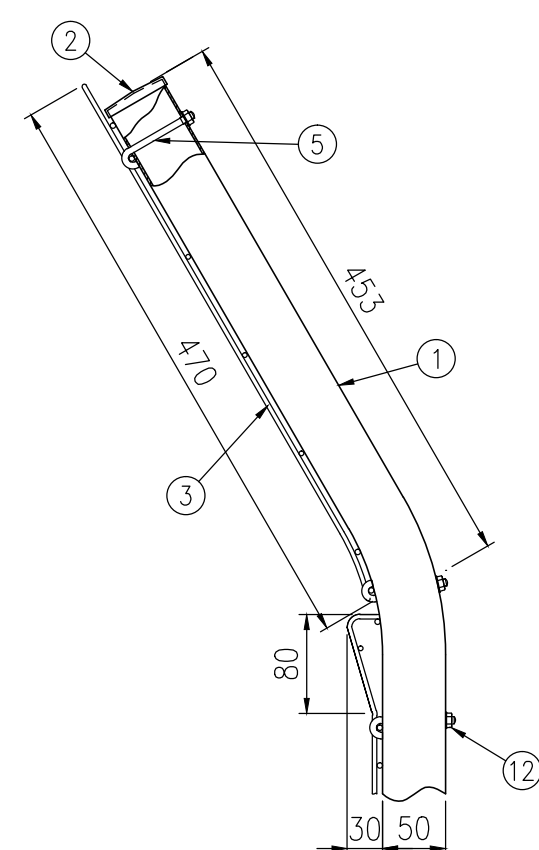
<外忍びの場合 取付部詳細図> (1/6)
