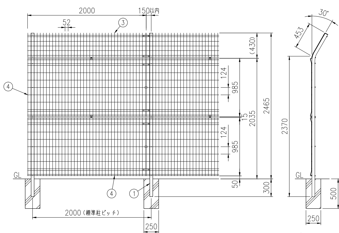
組立図 (1/30) 注) 基礎の大きさは参考寸法です。
