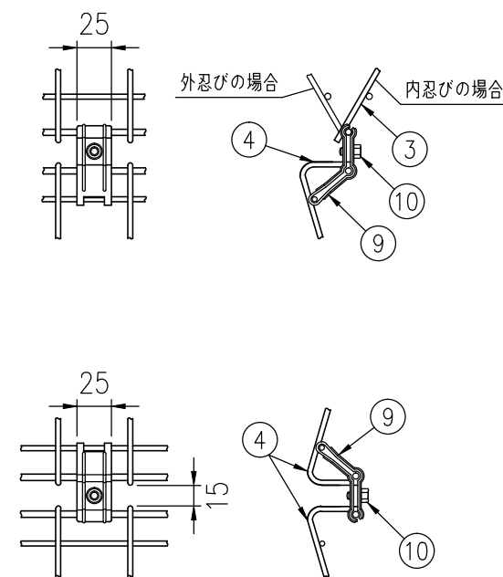
パネル上下連続金具詳細図 (1/5)
