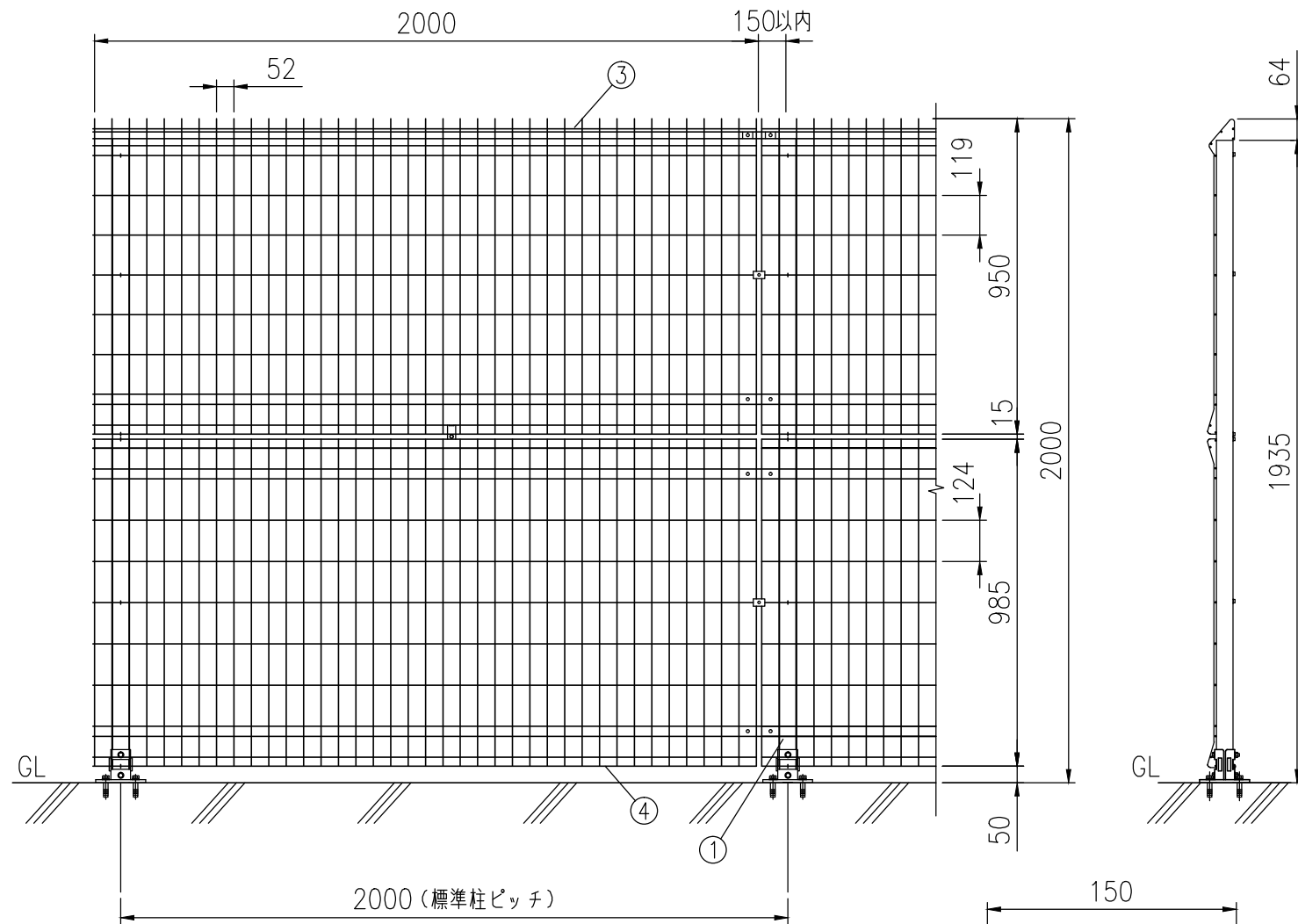
組立図 (1/20)
