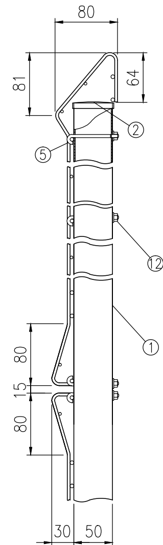
取付部詳細図 (1/5)
