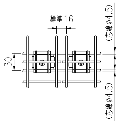
接続部詳細図 (1/5)
