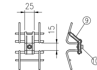
パネル上下連続金具詳細図 (1/5)
