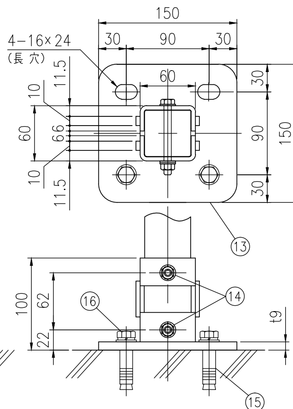
ベースプレート詳細図 (1/4)
