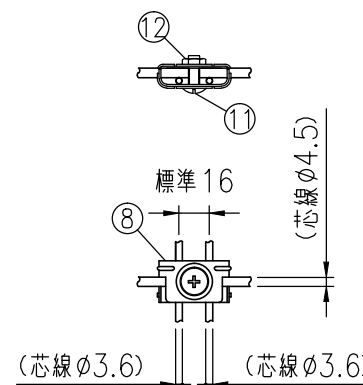
パネル止金具詳細図 (1/5)
