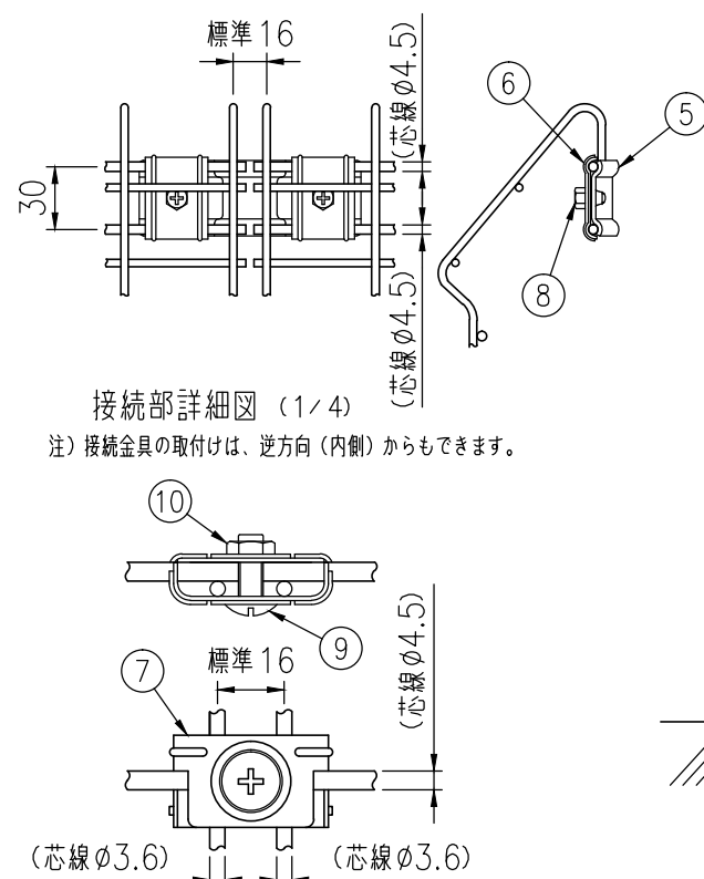
パネル止金具詳細図 (1/2) 注) パネル止金具の取付けは、逆方向(内側)からでもできます。
