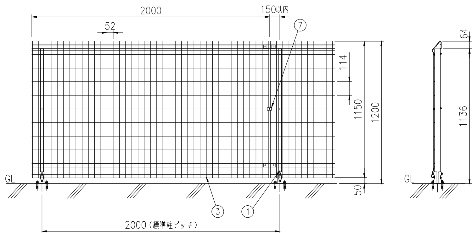
組立図 (1/20)
