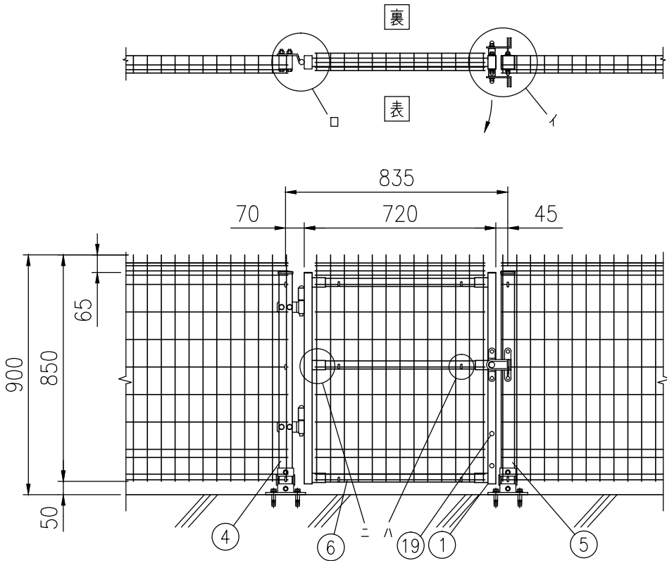
組立図 吊元が左、表開き（1/20） 注）基礎の大きさは参考寸法です。
