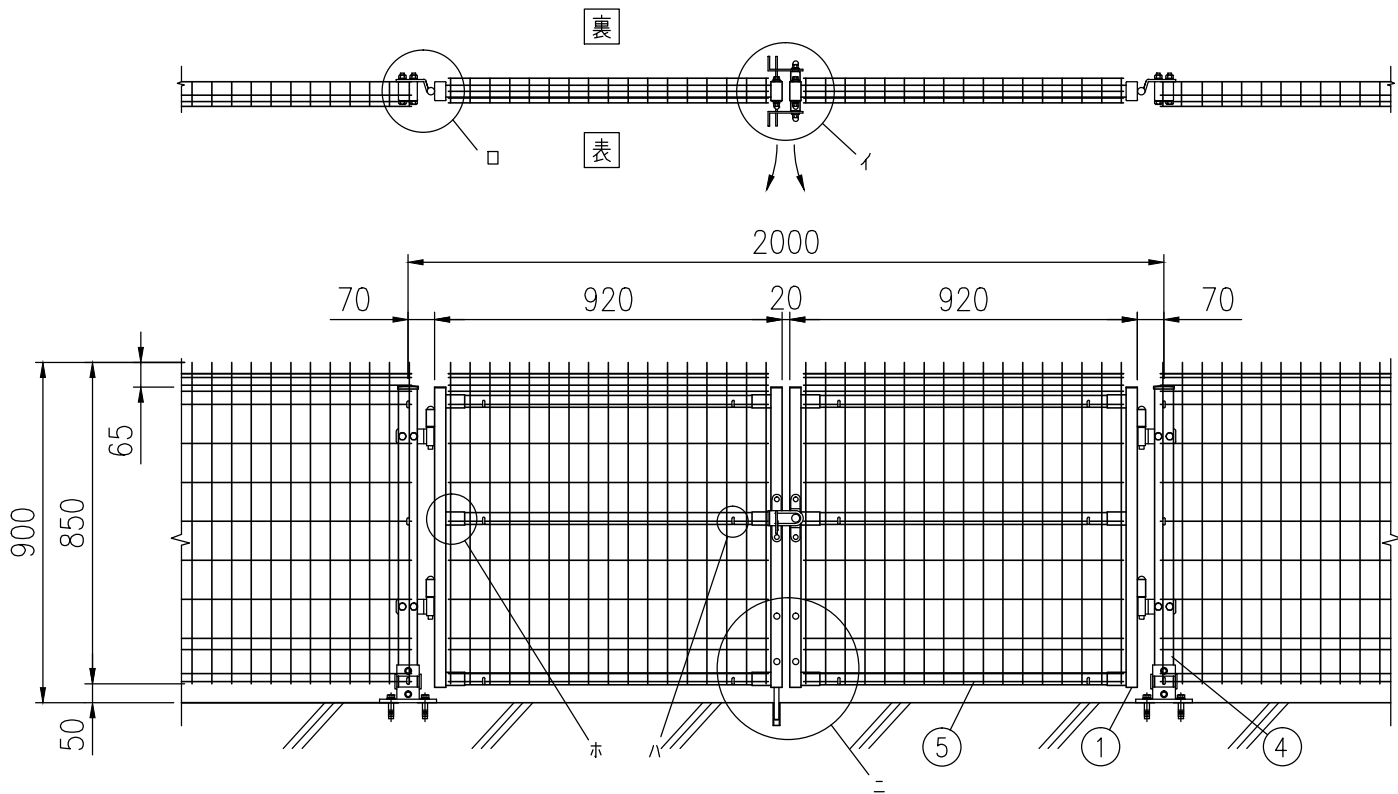
組立図 表開き、落とし棒が裏の時（1/20） 注>基礎の大きさは参考寸法です。
