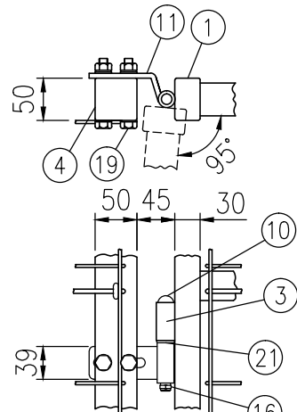
ロ部詳細図（1/8）
