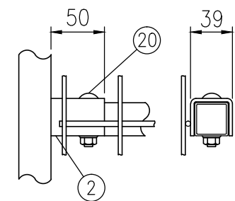
ホ部詳細図（1/5）
