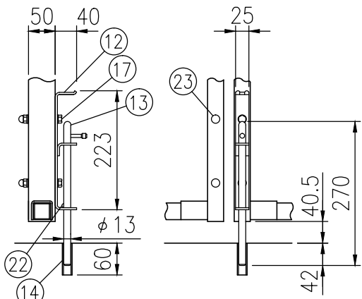
ニ部詳細図（1/10）
