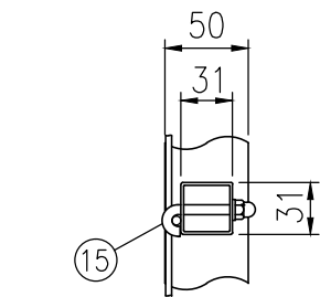
ハ部詳細図（1/5）
