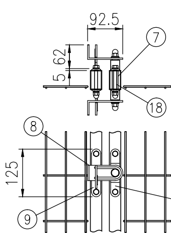
イ部詳細図（1/10）
