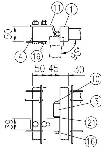
口部詳細図（1/8）
