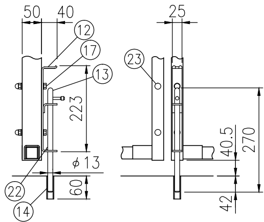
II部詳細図（1/10）
