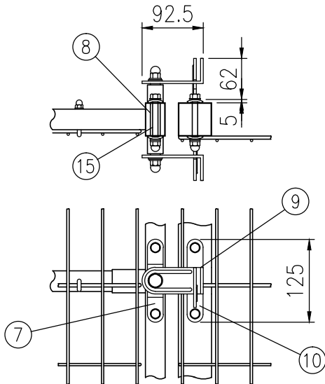
イ部詳細図（1/8）
