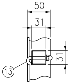
ハ部詳細図（1/5）
