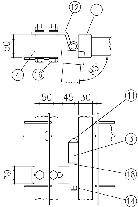
口部詳細図（1/5）
