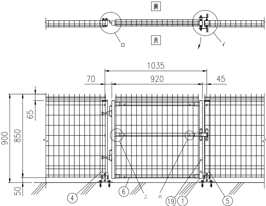
組立図 吊元が左、表開き（1/20） 注＞基礎の大きさは参考寸法です。
