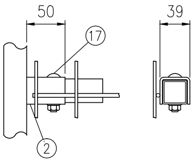
ニ部詳細図（1/5）
