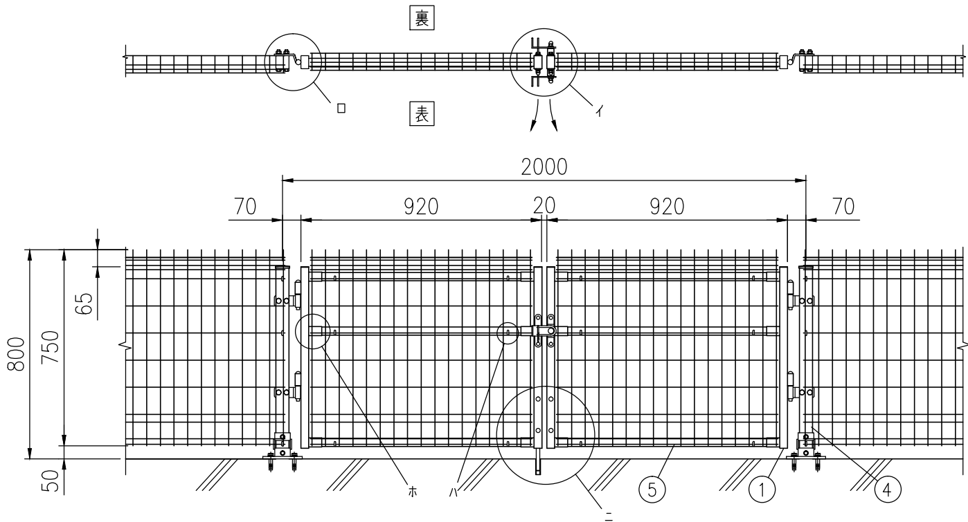
組立図 表開き、落とし棒が裏の時（1/20） 注>基礎の大きさは参考寸法です。
