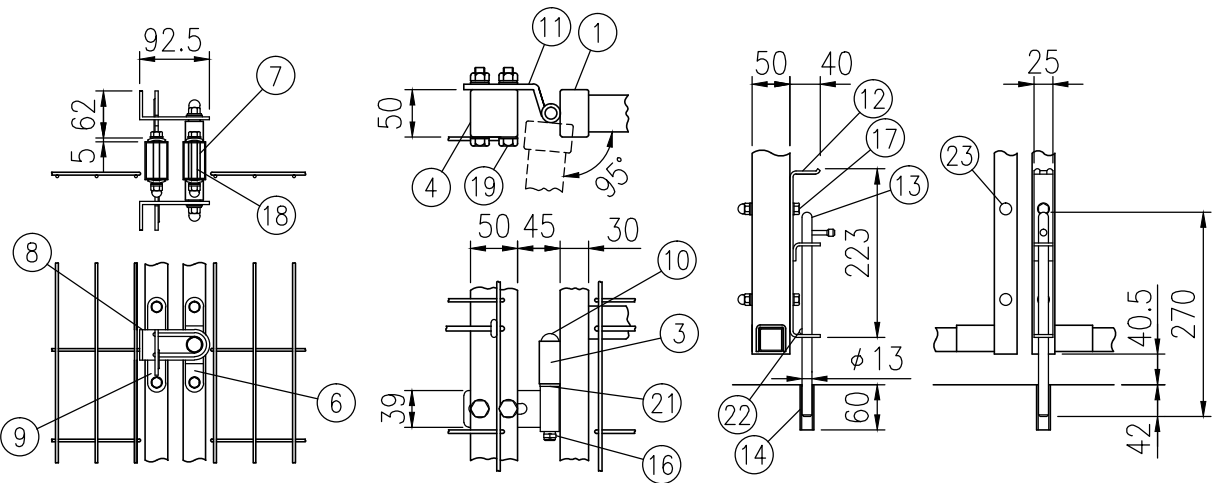
I部詳細図（1/10） ロ部詳細図（1/8） ニ部詳細図（1/10）
