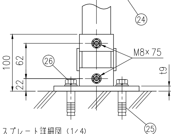
ベースプレート詳細図（1/4）
