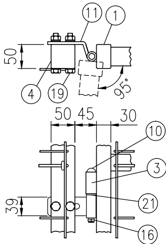
II部詳細図（1/8）
