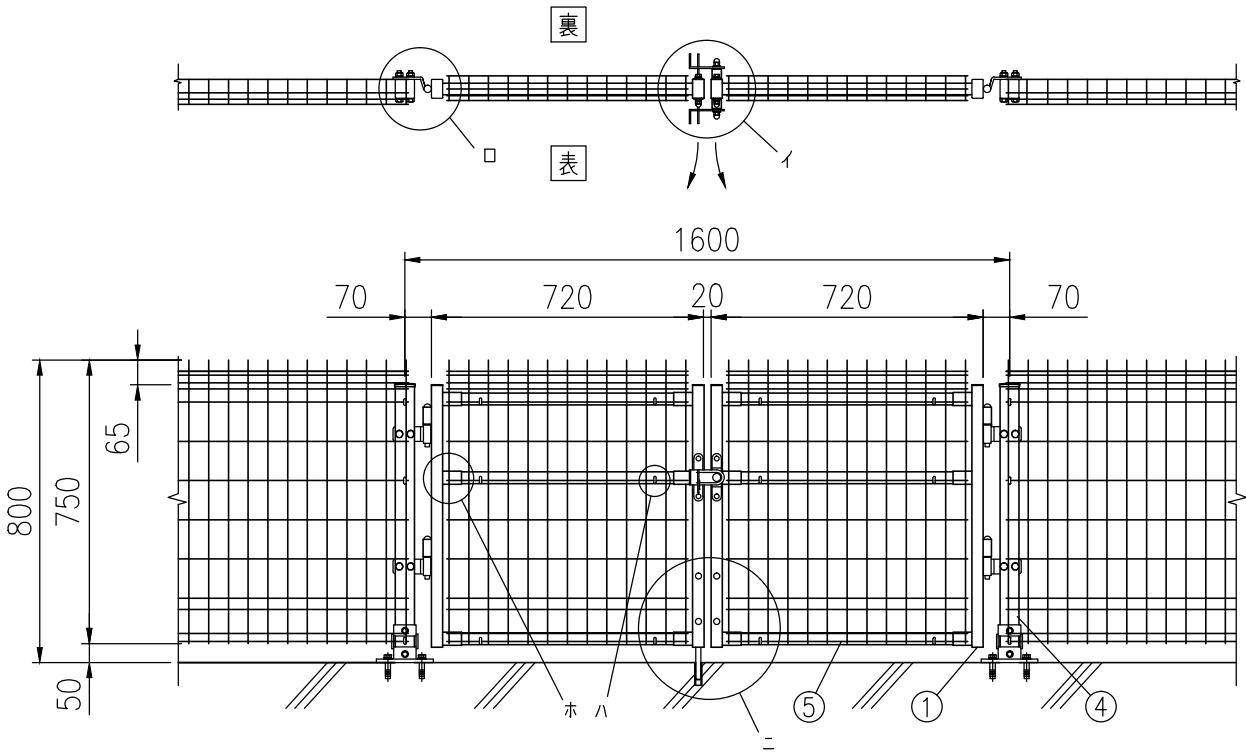
組立図 表開き、落とし棒が裏の時（1/20） 注＞基礎の大きさは参考寸法です。
