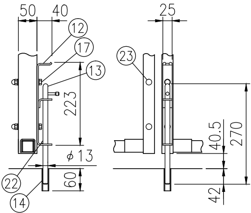
III部詳細図（1/10）
