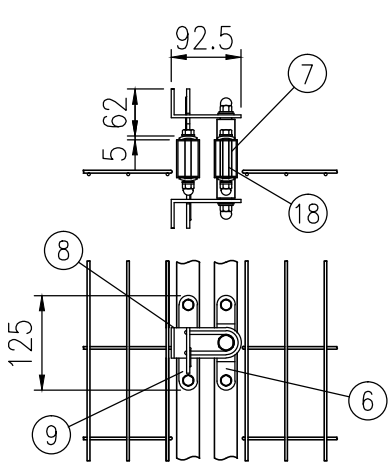
I部詳細図（1/10）
