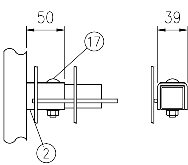
II部詳細図（1/5）
