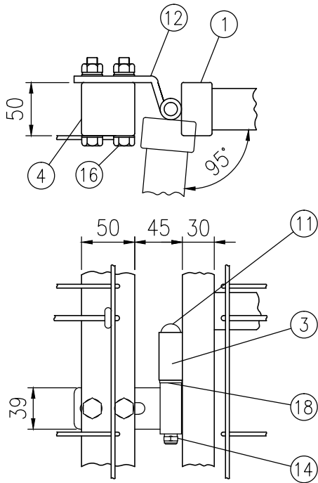
III部詳細図（1/5）
