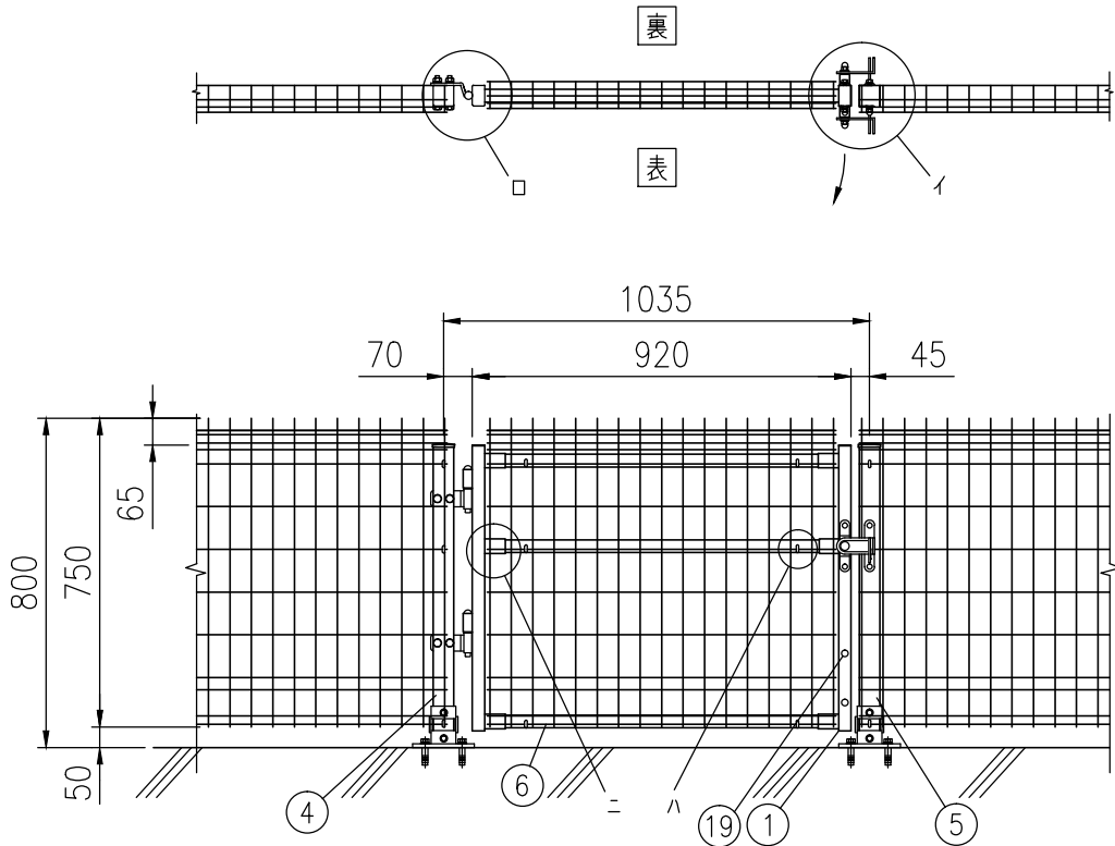
組立図 吊元が左、表開き（1/20） 注＞基礎の大きさは参考寸法です。
