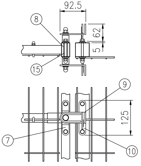
イ部詳細図 (1/8)
