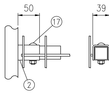
ニ部詳細図 (1/5)
