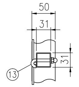
ハ部詳細図 (1/5)
