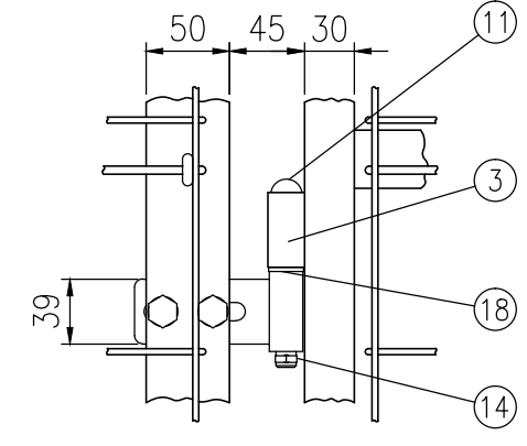
ロ部詳細図 (1/5)
